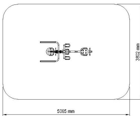
Strefa bezpieczeństwa dla urządzenia ST-013/ST-004
