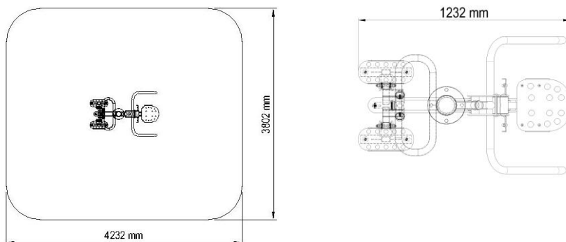
Strefa bezpieczeństwa dla urządzenia ST-022/ST-008
