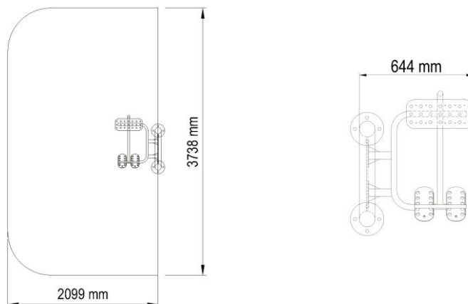
Strefa bezpieczeństwa dla urządzenia ST-020
