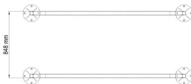
Strefa bezpieczeństwa dla urządzenia ST-024
