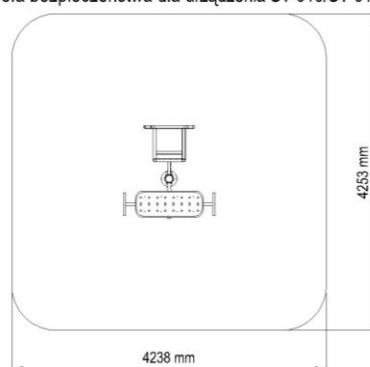
Strefa bezpieczeństwa dla urządzenia ST-010/ST-018
