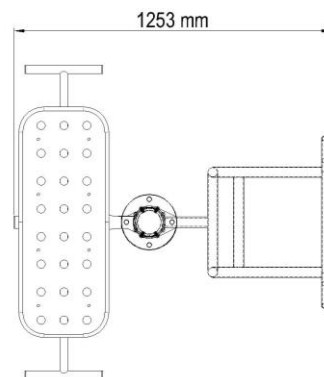
Strefa bezpieczeństwa dla urządzenia ST-010/ST-018
