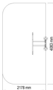
Strefa bezpieczeństwa dla urządzenia ST-027
