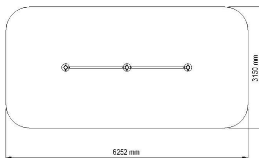
Strefa bezpieczeństwa dla urządzenia ST-027
