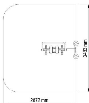
Strefa bezpieczeństwa dla urządzenia ST-005
